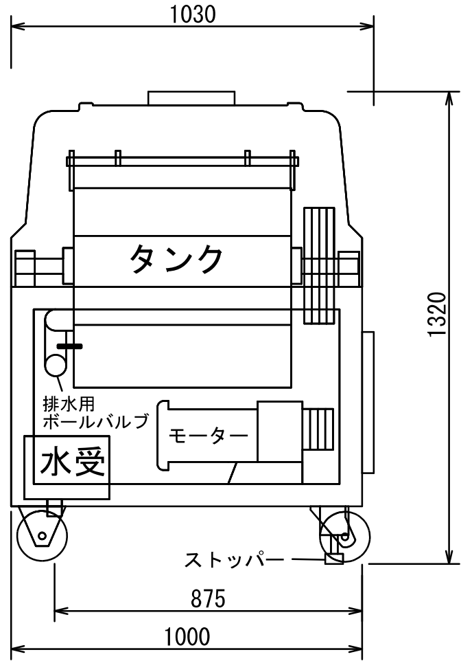
正面図
