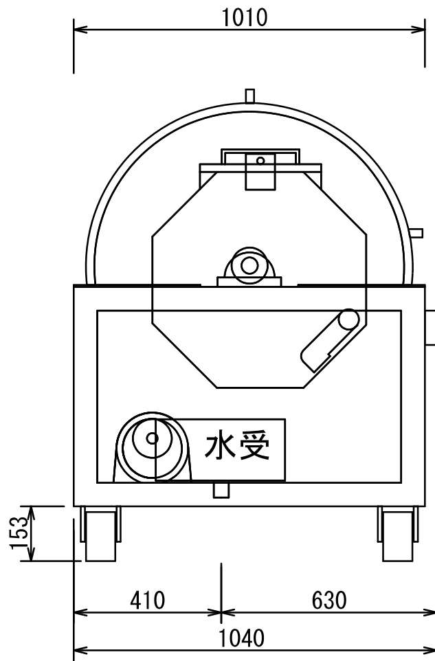
左側面図
